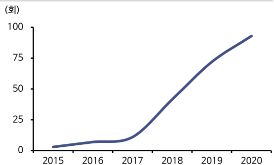
관측 가능한 중력파 횡수 누적 추이
